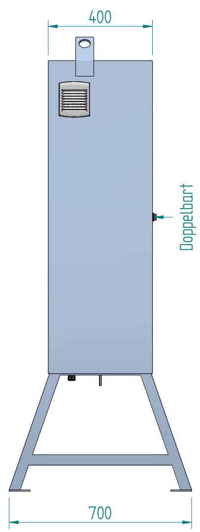
Schema Art.Nr. 229297
