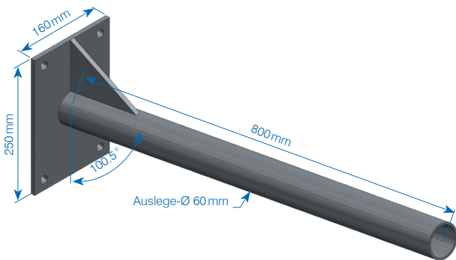
Wandausleger Art.-Nr. 136695
