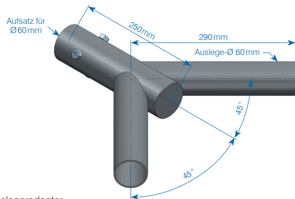
Auslegeradapter Art.-Nr. 137727
