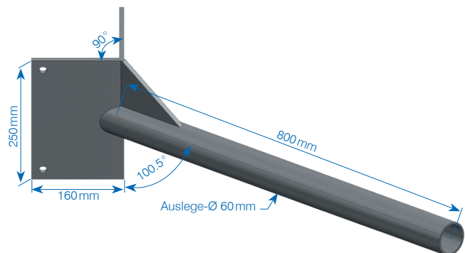
Eckausleger Art.-Nr. 137688
