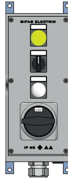
Typ 2812 120×268×132 mm
