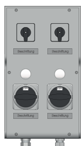
Typ 7350 200×350×133 mm
