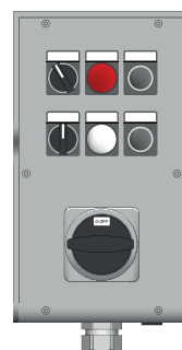
Typ 7250 160×280×133 mm
