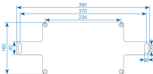
Montageplatte quer V4A rostfrei zu Dosen Typ 2516 Art. Nr. 207052
