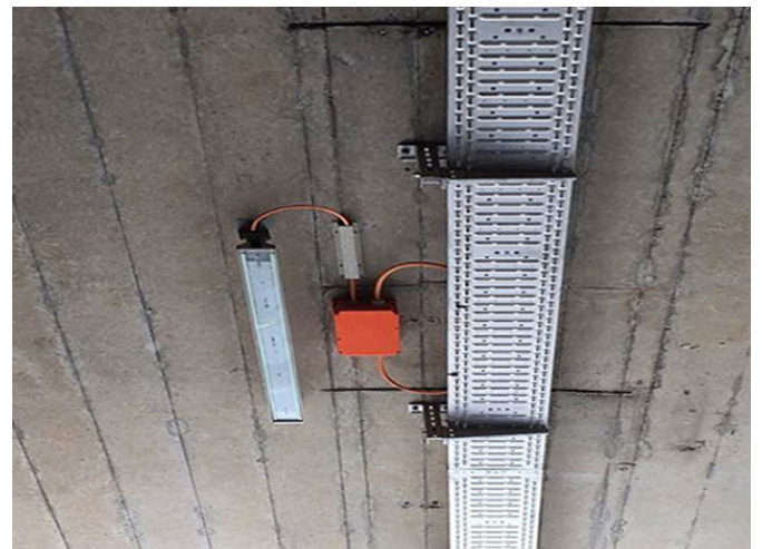
Typisches Beispiel einer Installation mit Adaption Beleuchtung für Not Netz in FE180/E30
